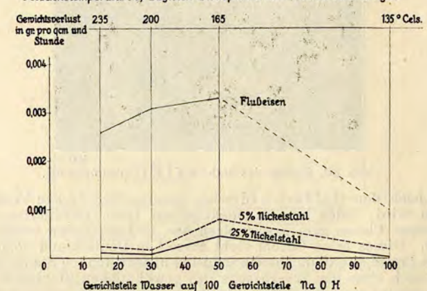
Abb. 18. Widerstandsfähigkeit gegen Laugen.
