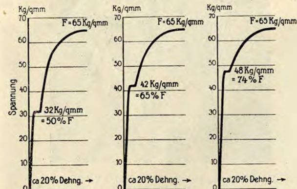
Abb. 14. Von links nach rechts: Spannungs-Dehnungsdiagramme eines Kohlenstoffstahls, eines Manganstahls und eines Chromnickelstahls.
