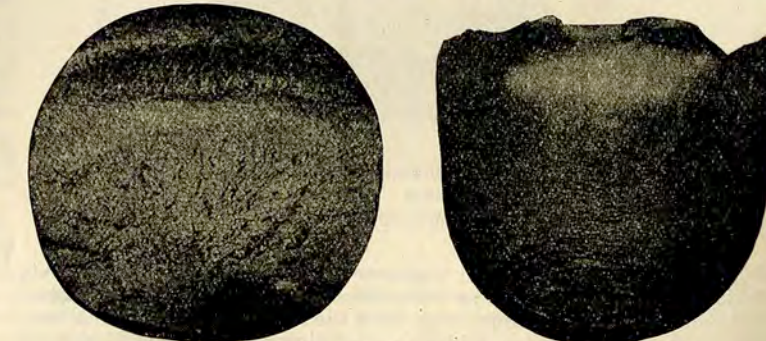
Abb. 13. Links: Rohbruch eines geglähten Martinstahls; rechts: Rohbruch eines vergüteten 5%igen Nickelstahls. (Die Stücke hatten in Wirklichkeit einen Durchmesser von 200 mm.)
