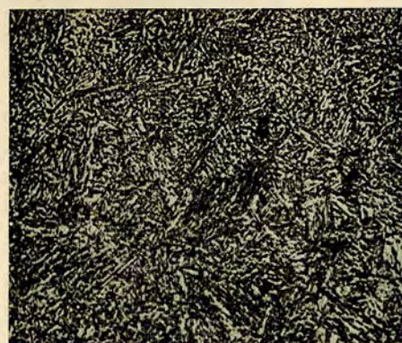
Abb. 6. Martensit eines langsam erkalteten 12%igen Nickelstahls.
