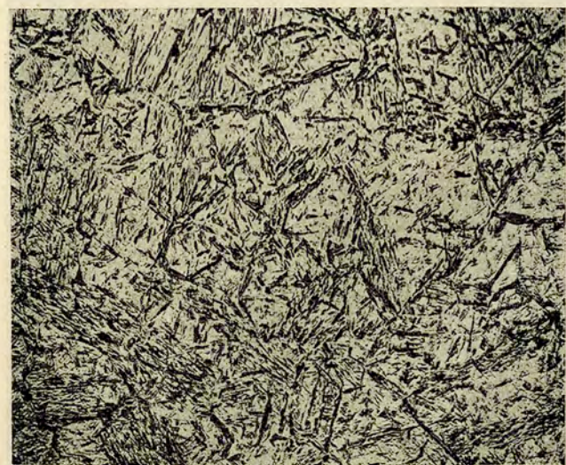
Abb. 5. Martensit der Randzone eines in Wasser gehärteten Kohlenstoffstahls.
