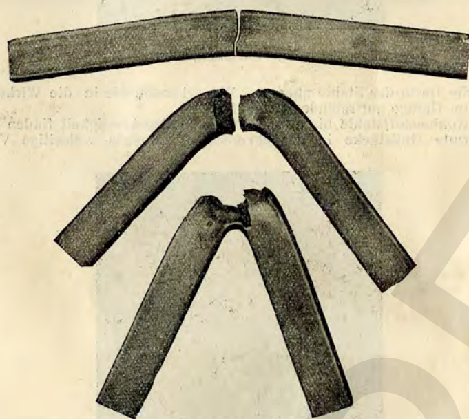
Abb. 16. Gekerbte Biegeproben aus denselben Stählen. Oben: Kohlenstoffstahl; Mitte: Manganstahl; unten: Chromnickelstahl.
