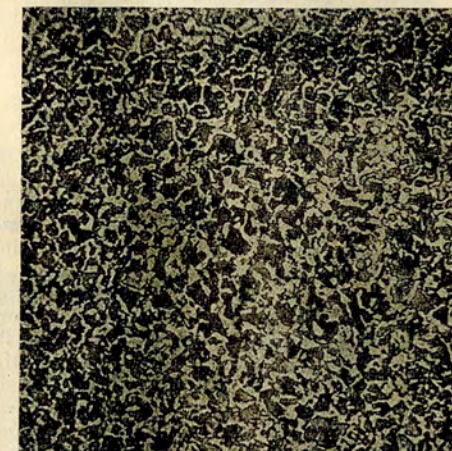
Abb. 2. Stahl mit 0,5% Kohlenstoff, gegläht. 100 ×
