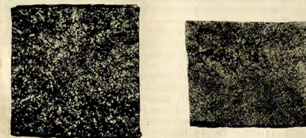
Abb. 10. Links: Rohbruch von ungeglühtem Stahlguß; rechts: Rohbruch von geglähtem Stahlguß. (Beide Bilder sind auf etwa 1/5 der nat. Größe verkleinert.)
