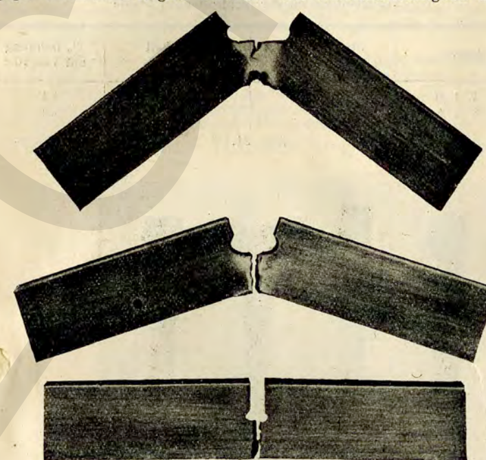
Abb. 17. Kerbschlagproben aus denselben Stählen. Oben: Chromnickelstahl mit einer Kerbzähigkeit von 28 mkg/qcm. Mitte: Manganstahl „ „ „ 12 „ „ „ „ „ 12 „ „ „ „ „ 4 „ „ „ „ „ 4 „ „
