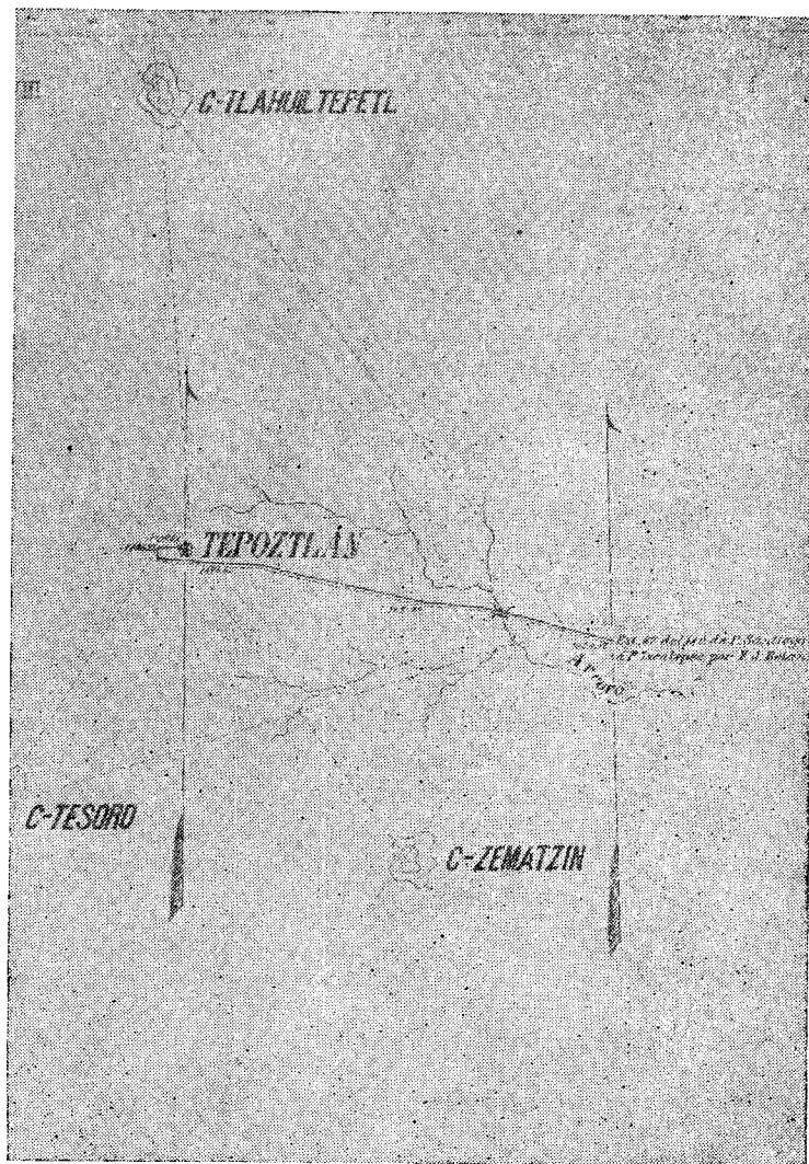
Fig. 7. Levantamiento planimétrico
